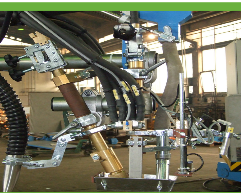
Glava za dubinsko zavarivanje do 250 mm - sa jednom žicom, tandem izvedba
