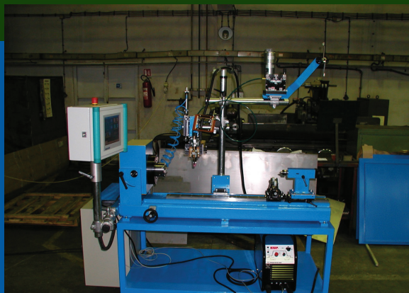
Uređaji za TIG zavarivanje
