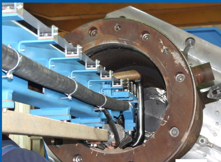
Glava za navarivanje pomoću trake – u izvedbi za navarivanje u zadanom promjeru i u izvedbi za otvorene mjere
